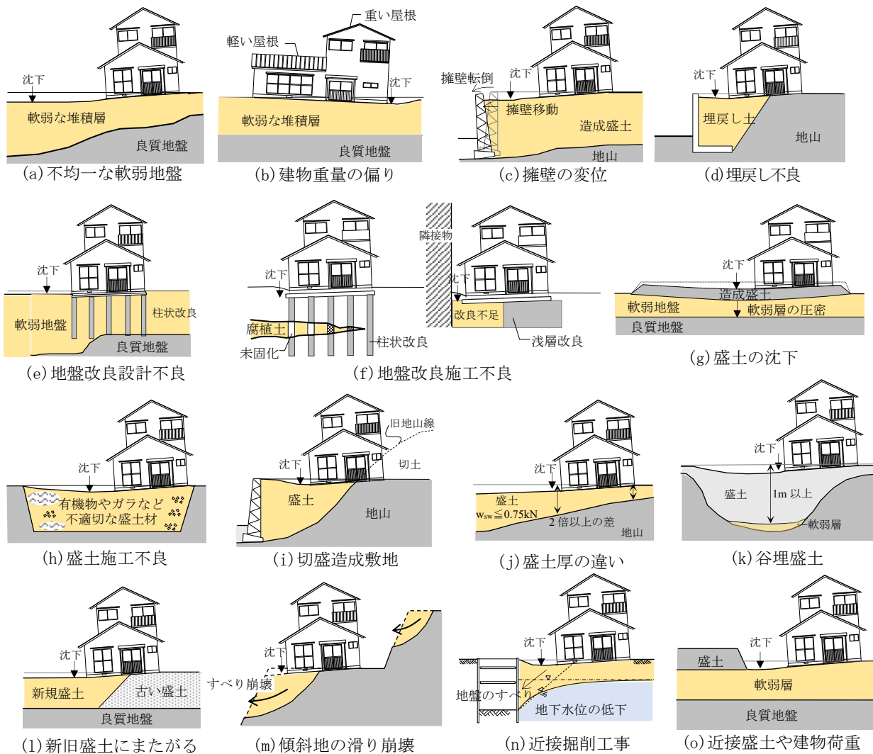
図-2 不同沈下の原因例
